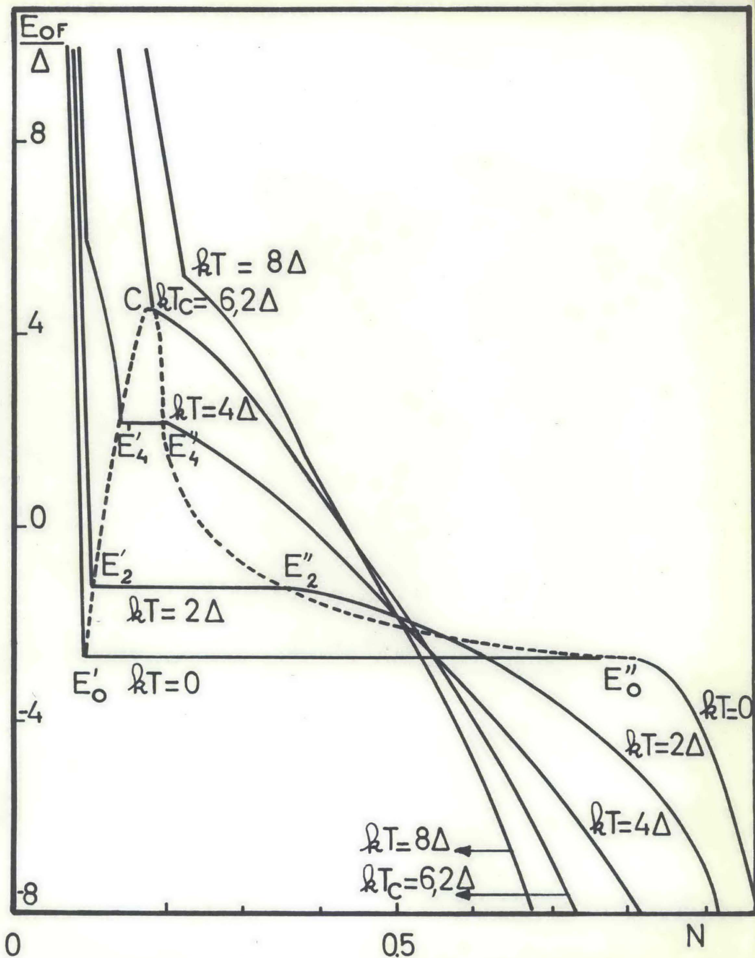
Fig-21: Nombre total d'électrons \frac{U}{\Delta} = 250 - \frac{J}{\Delta} = 150
